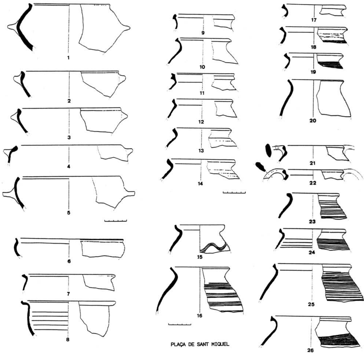
Lámina 1: Contextos cerámicos (ss. V-VI) de la Pl. de Sant Miquel (Barcelona). (Dibujo de Jordi Roig i Buxó, 1995).
